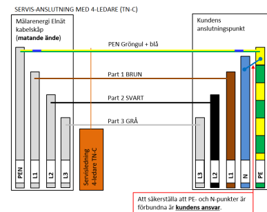
Anslutningsschema av servisledning
