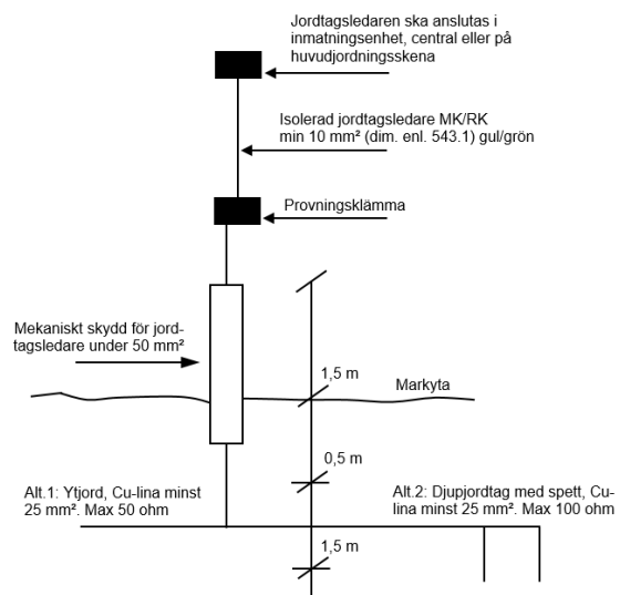
Jordningsutförande
