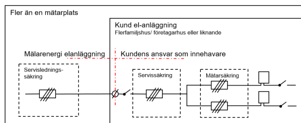
Mätarplats för fler än en mätare
