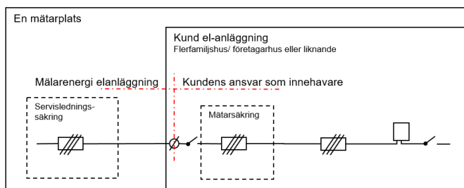
Mätarplats för en mätare
