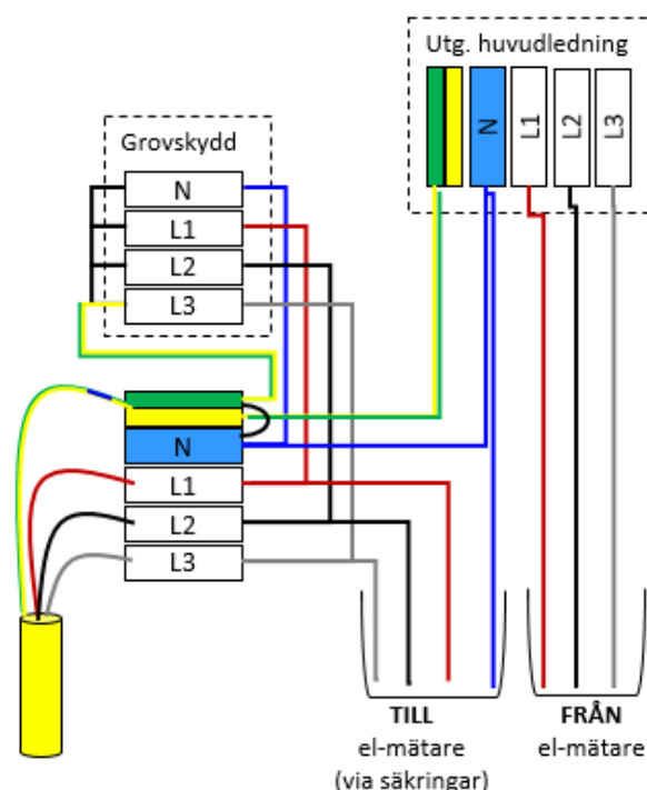
3.4 Schematisk bild av överspänningsskyddets placering
