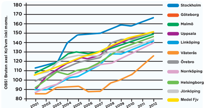
Fjärrvärmepriser i landets tio största kommuner över perioden 2001-2012.
